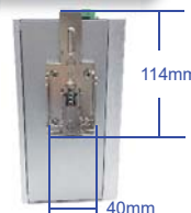
DIN Rail Mount Kit
