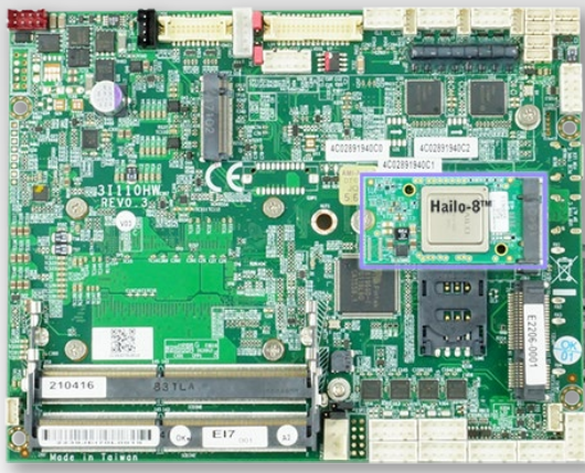
31110HW/BW + Hailo-8™ AI module
