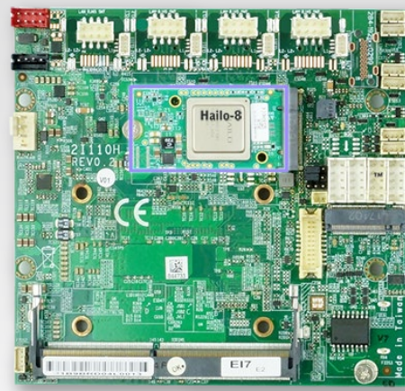
21110H + Hailo-8™ AI module
