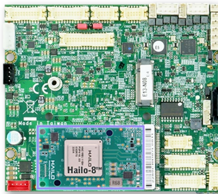
21640HW + Hailo-8™ AI module
