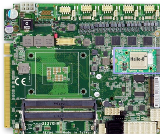
31370HW + Hailo-8™ AI module
